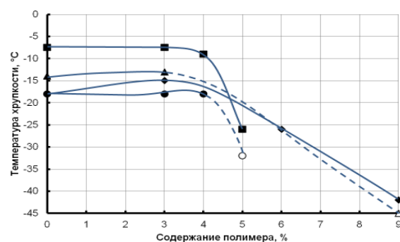
Рис. 1. Изменение температуры хрупкости БМП при повышении концентрации полимера типа СБС при использовании битумов: \diamond – Бм1, \blacktriangle – Бм2, \blacksquare – Бо, \bullet – Би; светлыми маркерами показаны пределы, ниже которых находится температура хрупкости соответствующего вяжущего
