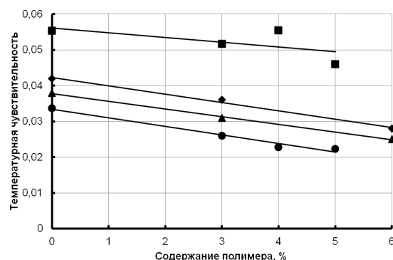
Рис. 2. Изменение температурной чувствительности вяжущего при модификации полимером типа СБС битумов: \diamond – Бм1, \blacktriangle – Бм2, \blacksquare – Бо, \bullet – Би
